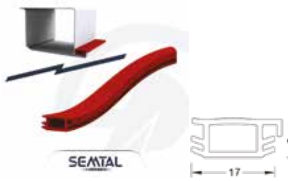
Yangın Grubu Contası Fire Group Wick SMP-20112
